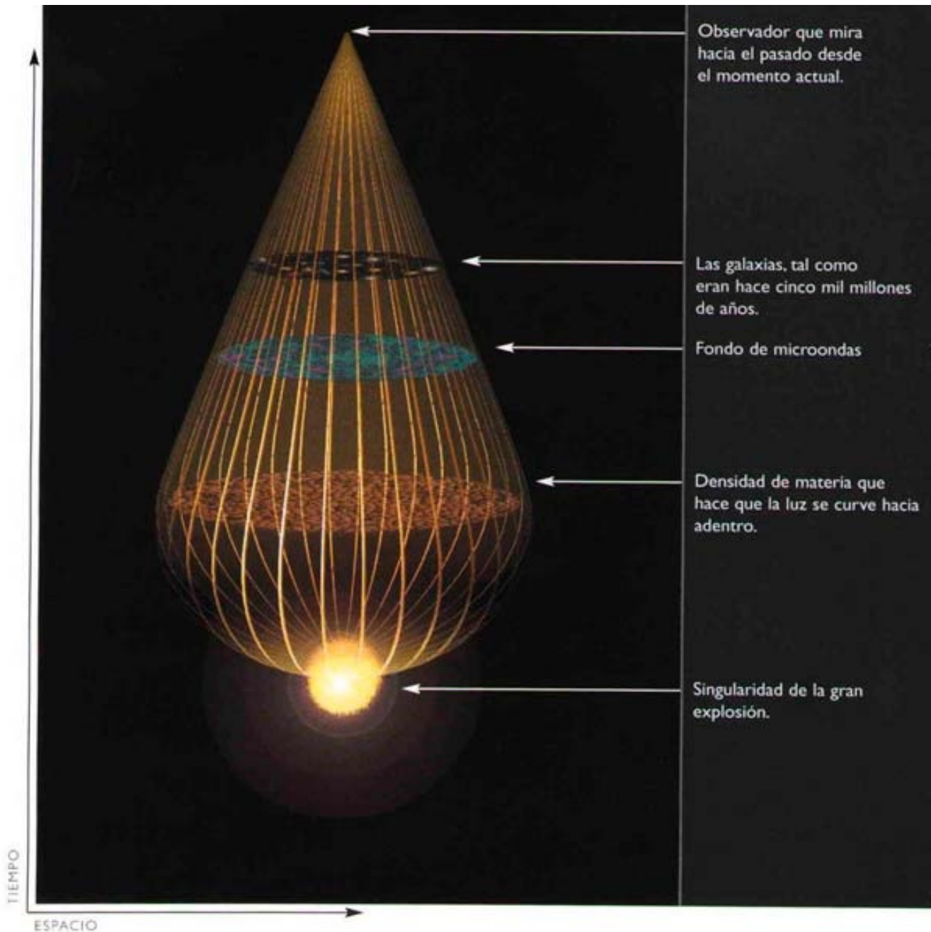
(FIG. 2.8) EL TIEMPO TIENE FORMA DE PERA
