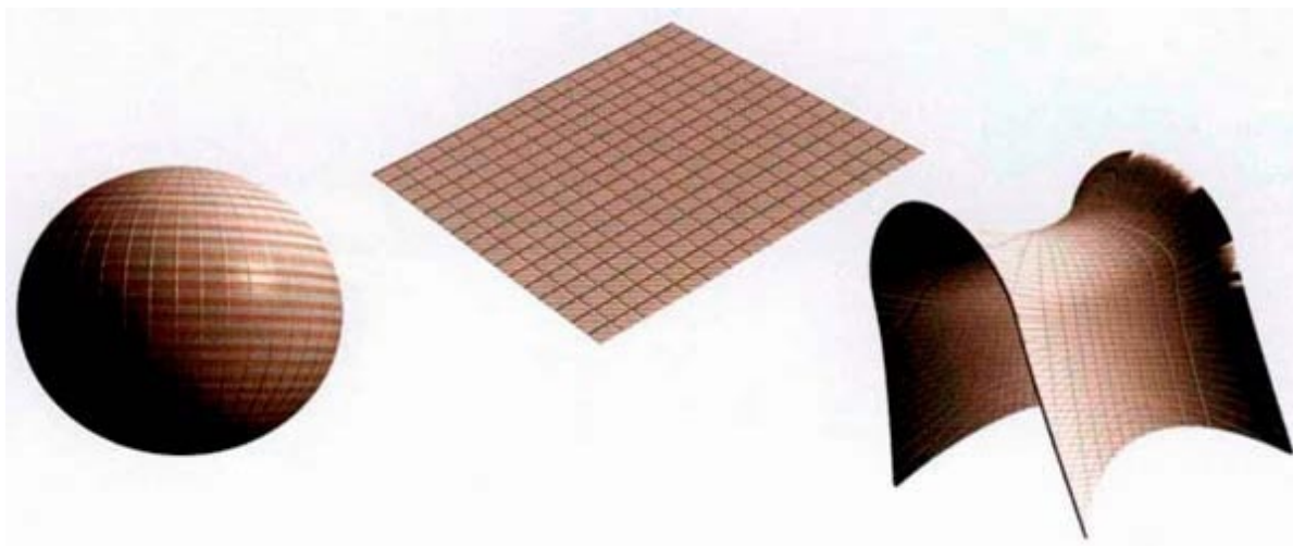
(FIG. 3.9) HISTORIAS DEL UNIVERSO
