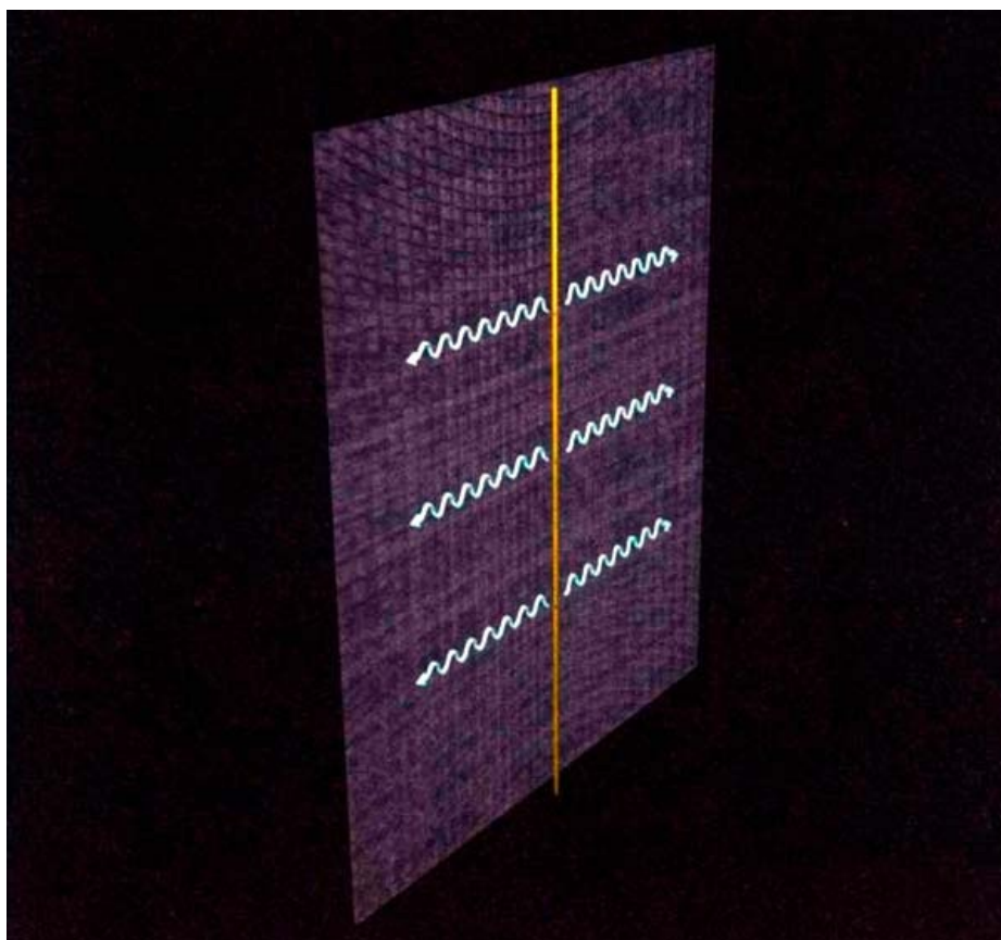
(FIG. 7.7) UNIVERSOS MEMBRANA
