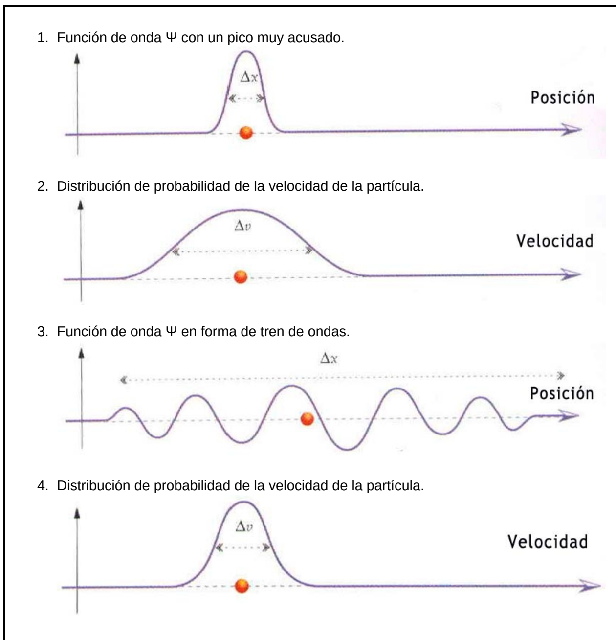
(FIG. 4.4) La función de onda determina las probabilidades de que la partícula se halle en diferentes posiciones y tenga diferentes velocidades, de forma que \Delta x y \Delta v obedezcan en principio de incertidumbre.
