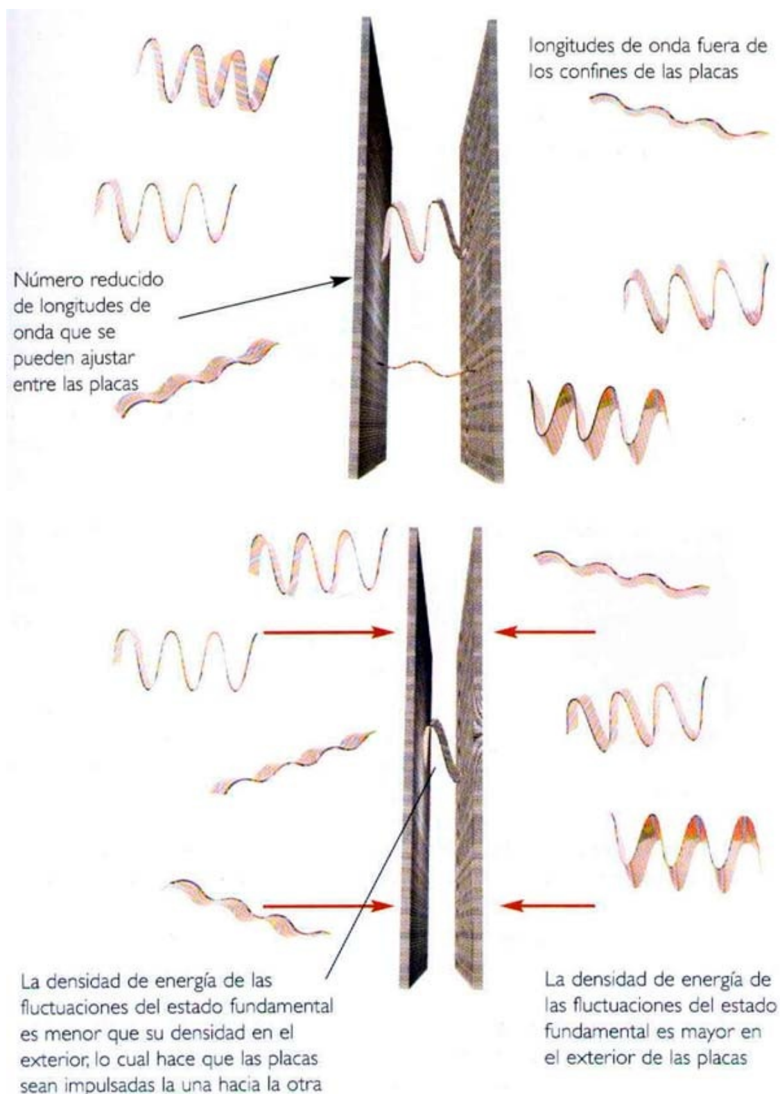
(FIG. 2.11) EFECTO CASIMIR
