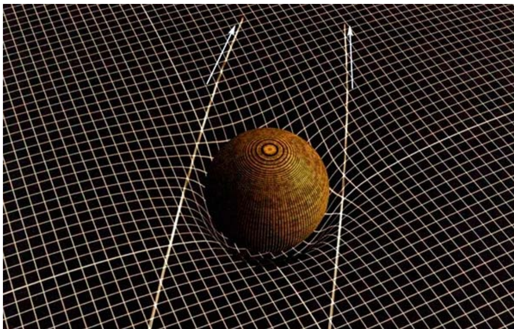
(FIG. 2.7) DEFORMANDO EL ESPACIO-TIEMPO
