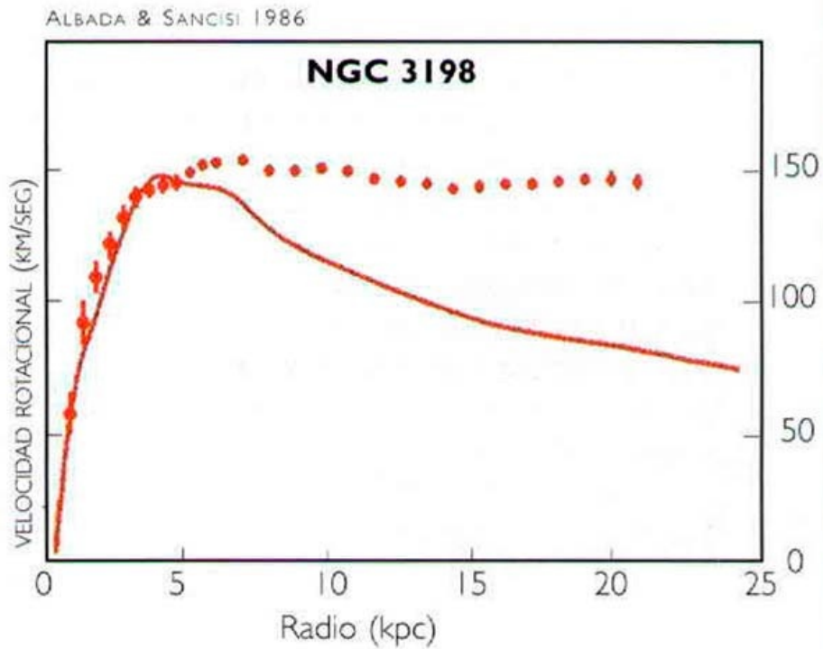
CURVA DE ROTACIÓN DE LA GALAXIA ESPIRAL NGC 3198
