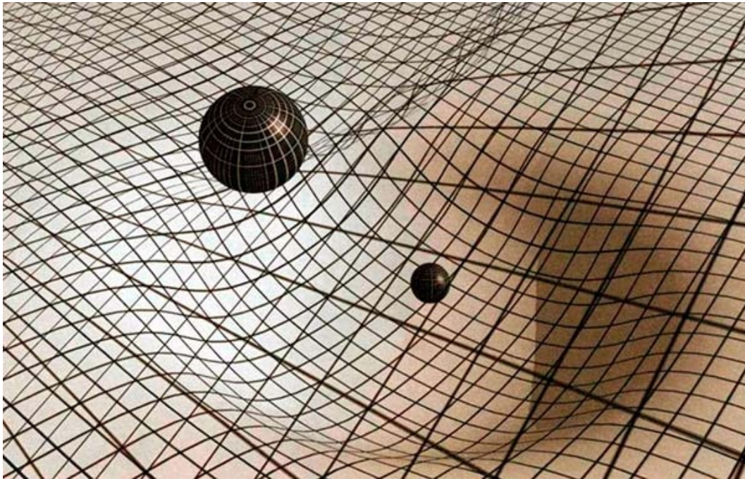
(FIG. 1.12) EL ESPACIO-TIEMPO SE CURVA
