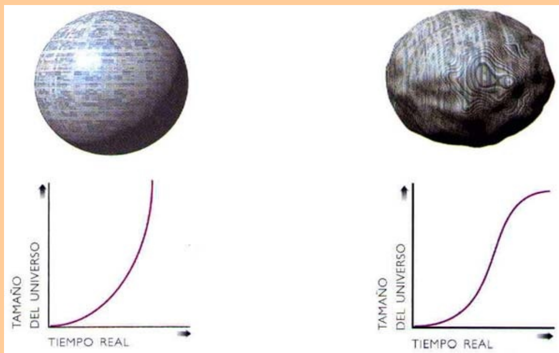
(FIG. 3.15) EL UNIVERSO INFLACIONARIO
