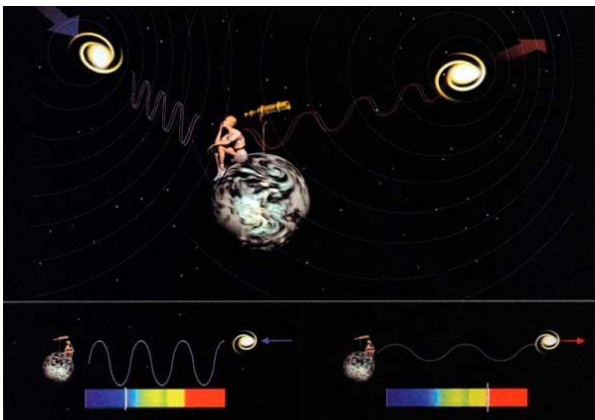
(FIG. 3.5) El efecto Doppler también se satisface para las ondas luminosas. Si una galaxia se mantuviera a una distancia constante de la Tierra, las líneas características de su espectro aparecerían en ciertas posiciones normales o estándar. Pero si la galaxia se está separando de nosotros, las ondas parecerán alargadas o estiradas y las líneas características se desplazarán hacia el rojo ( derecha ). Si la galaxia se nos está aproximando, parecerá que las ondas estén comprimidas, y las líneas estarán desplazadas hacia el azul ( izquierda ).
