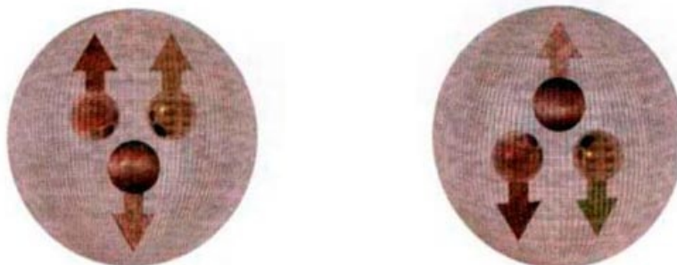
(FIG. 7.3) Izquierda: Un protón está formado por dos quarks arriba , cada uno de ellos con dos tercios de carga eléctrica positiva, y un quark abajo , con un tercio de carga eléctrica negativa. Derecha: Un neutrón está formado por dos quarks abajo , cada uno con un tercio de carga eléctrica negativa, y un quark arriba , con dos tercios de carga eléctrica positiva.
