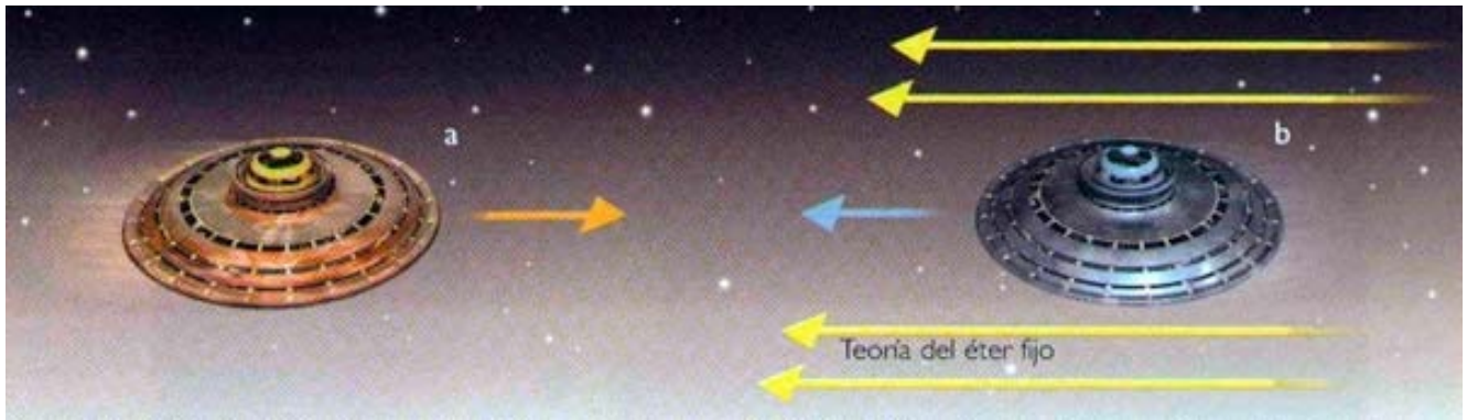
(FIG. 1.1) TEORÍA DEL ÉTER FIJO
