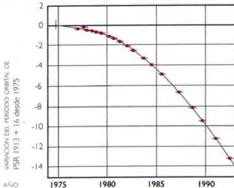
Gráfica del pulsar binario PSR1913+16 desde 1975
