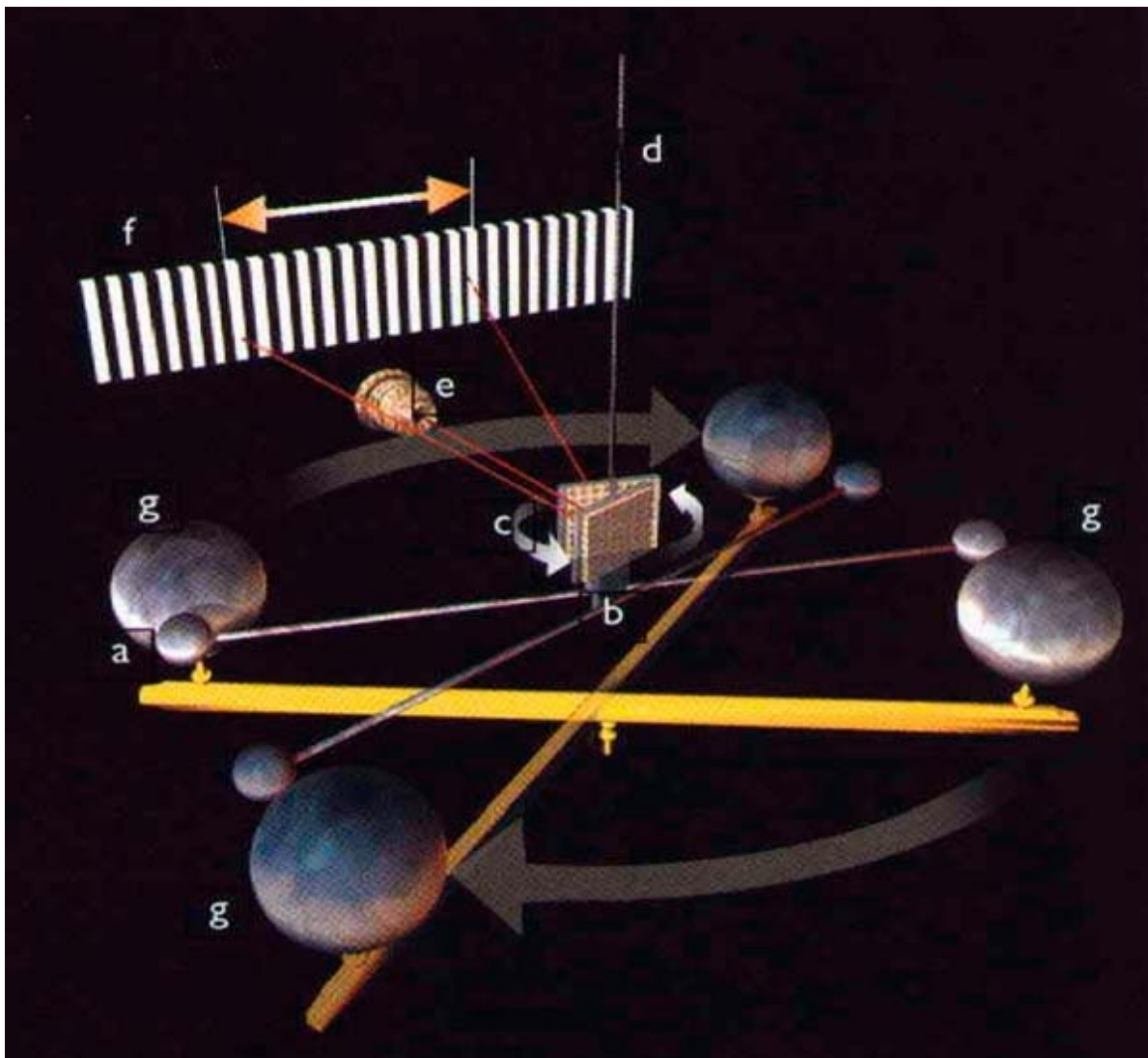
(FIG. 7.11) EL EXPERIMENTO DE CAVENDISH
