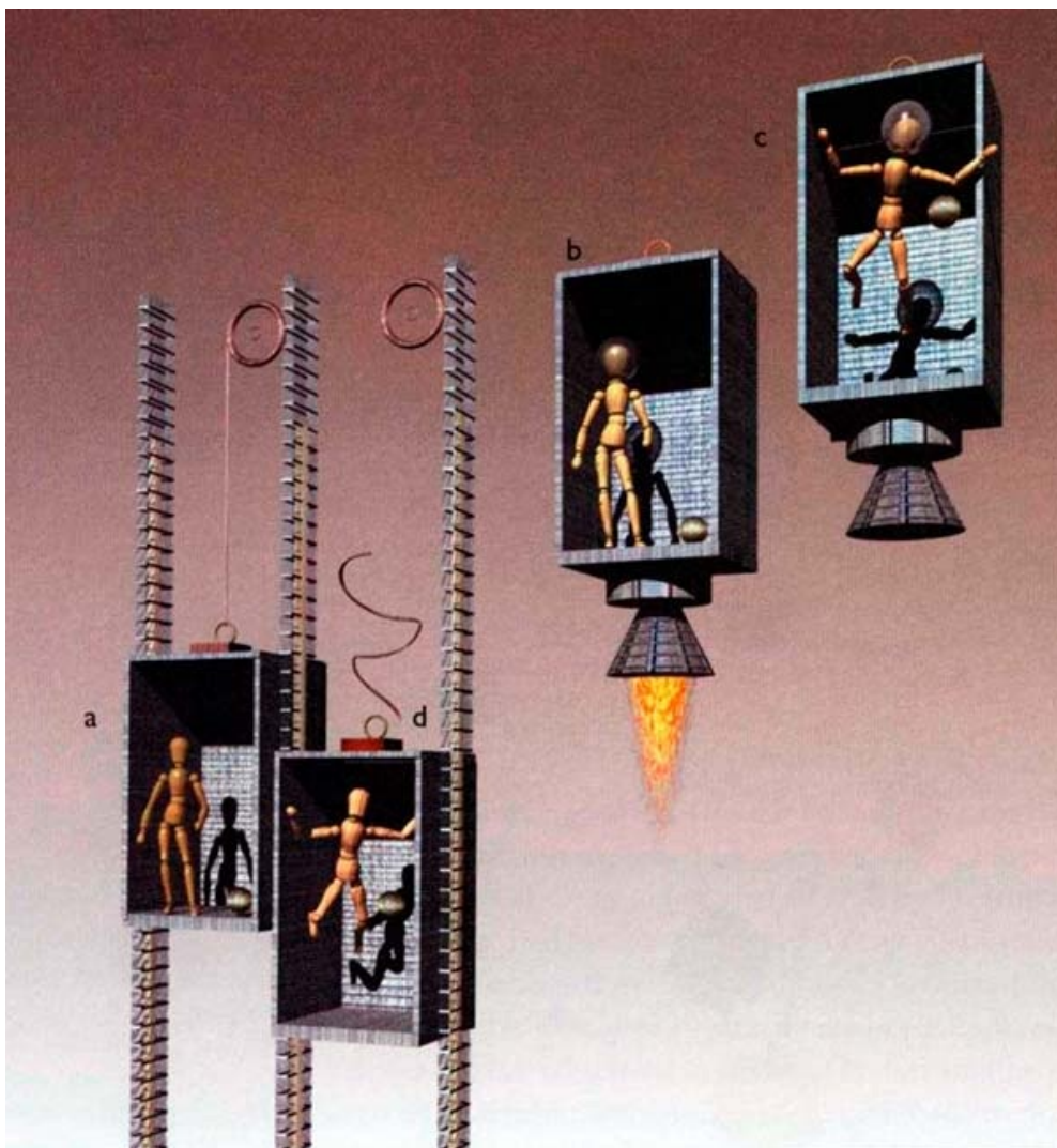
(FIG. 1.9) Un observador en una caja no puede notar la diferencia entre estar en un ascensor parado en la Tierra (a) o estar acelerado en un cohete en el espacio libre (b) .
