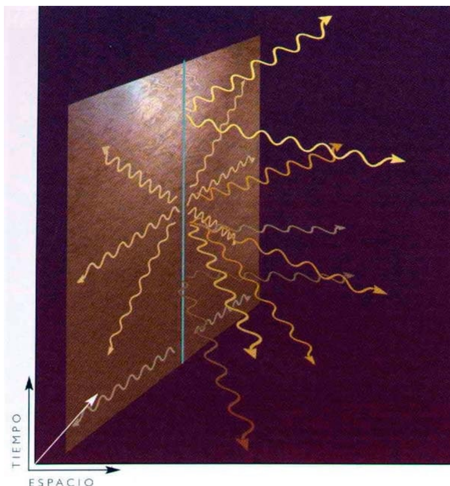
(FIG. 7.8) Además de actuar en la membrana, la gravedad se esparciría por las dimensiones adicionales y, por ello, disminuiría con la distancia más rápidamente que en el espacio-tiempo cuatridimensional.
