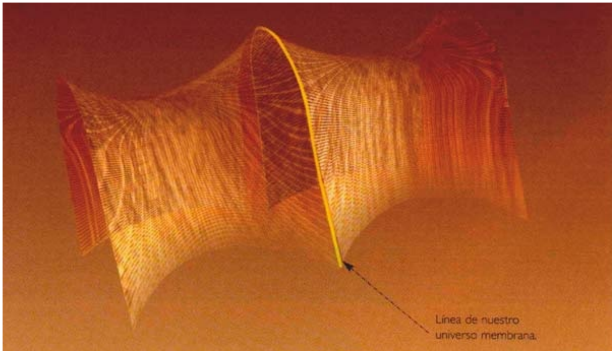
(FIG. 7.14) En el modelo de Randall-Sundrum sólo hay una membrana (mostrada aquí en una sola dimensión). Las dimensiones adicionales se extenderían hasta el infinito, pero estarían curvadas en forma de silla de montar. Esta curvatura impide que el campo gravitatorio de la materia situada en la membrana llegue hasta lejos en las dimensiones adicionales.
