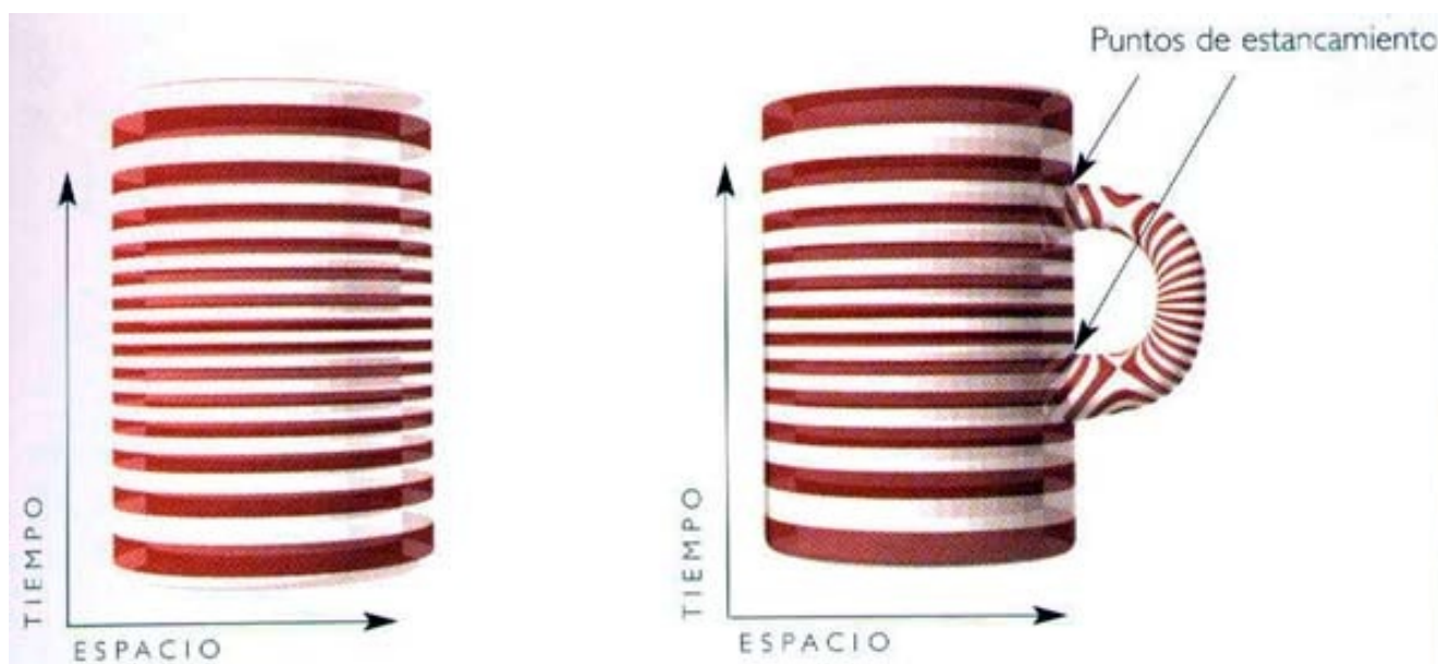
(FIG. 4.7) EL TIEMPO SE DETIENE
