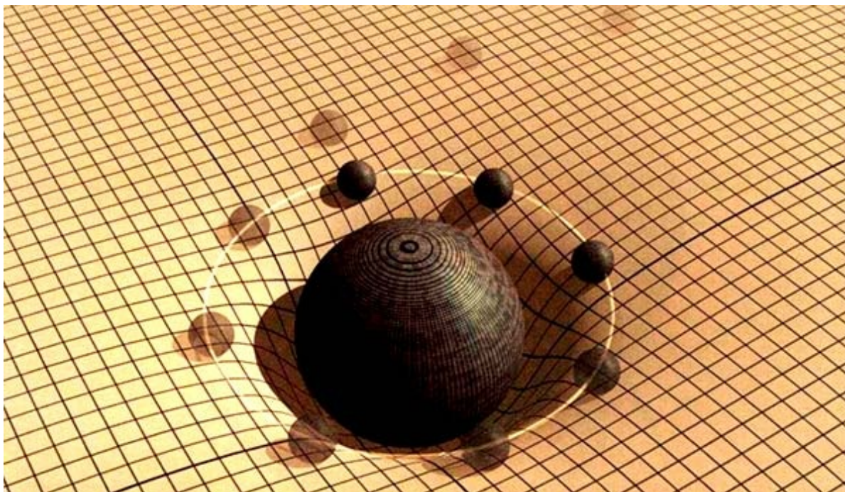
(FIG. 2.4) ANALOGÍA DE LA LÁMINA DE GOMA
