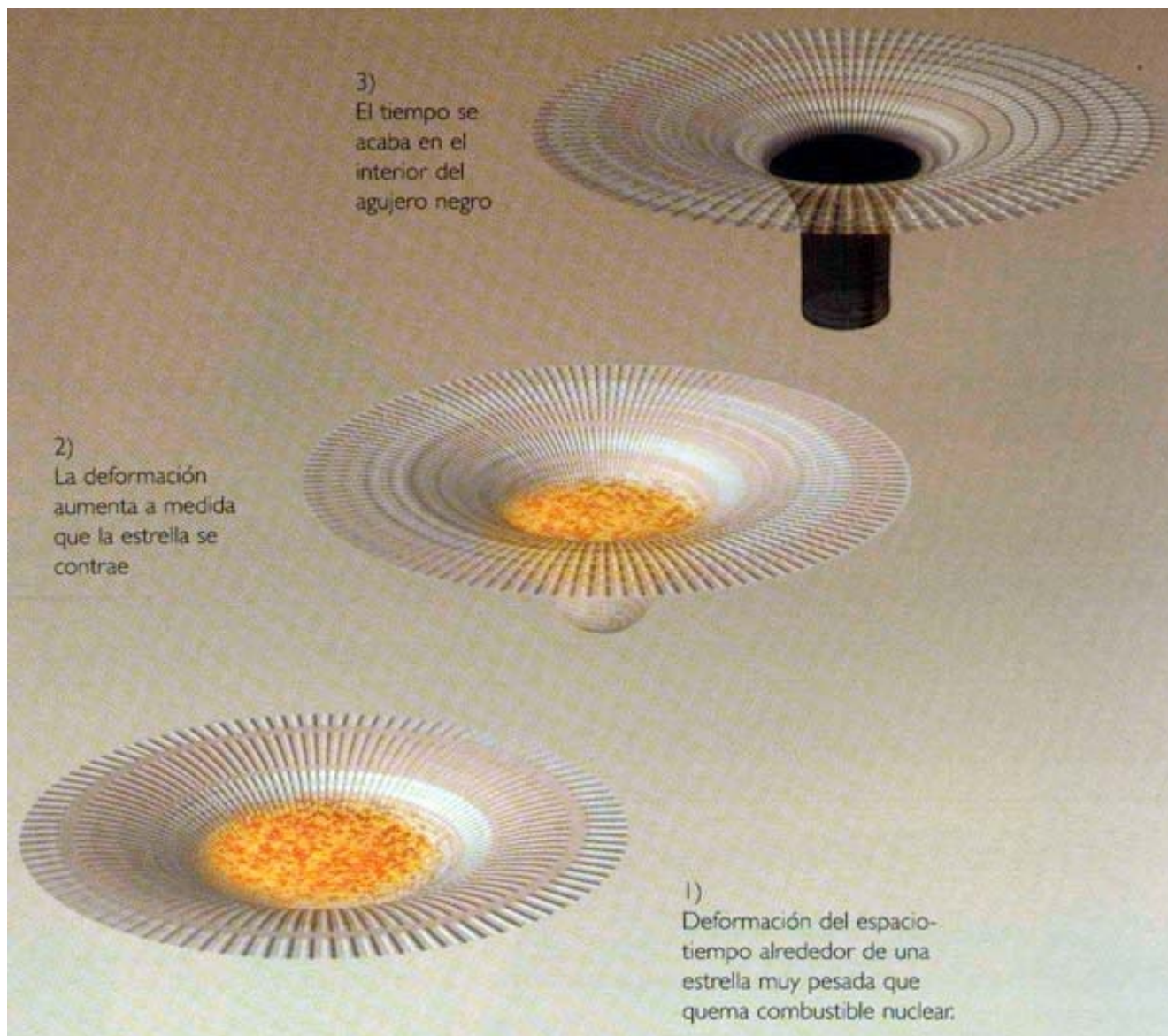
(FIG. 1.15) Cuando una estrella muy pesada agota su combustible nuclear, pierde calor y se contrae. La deformación del espacio-tiempo se hace tan grande que se forma un agujero negro, del cual la luz no puede escapar. En el interior del agujero negro el tiempo llega a su fin.
