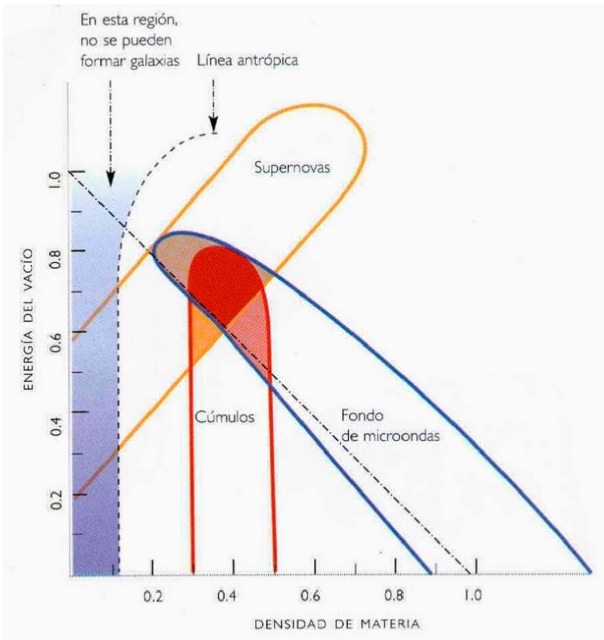
(FIG. 3.20) Combinando observaciones de supernovas distantes, de la radiación cosmica del fondo de microondas, y de la distribución de materia en el universo, podemos evaluar bastante bien la energía de vacío y la densidad de materia en el universo.
