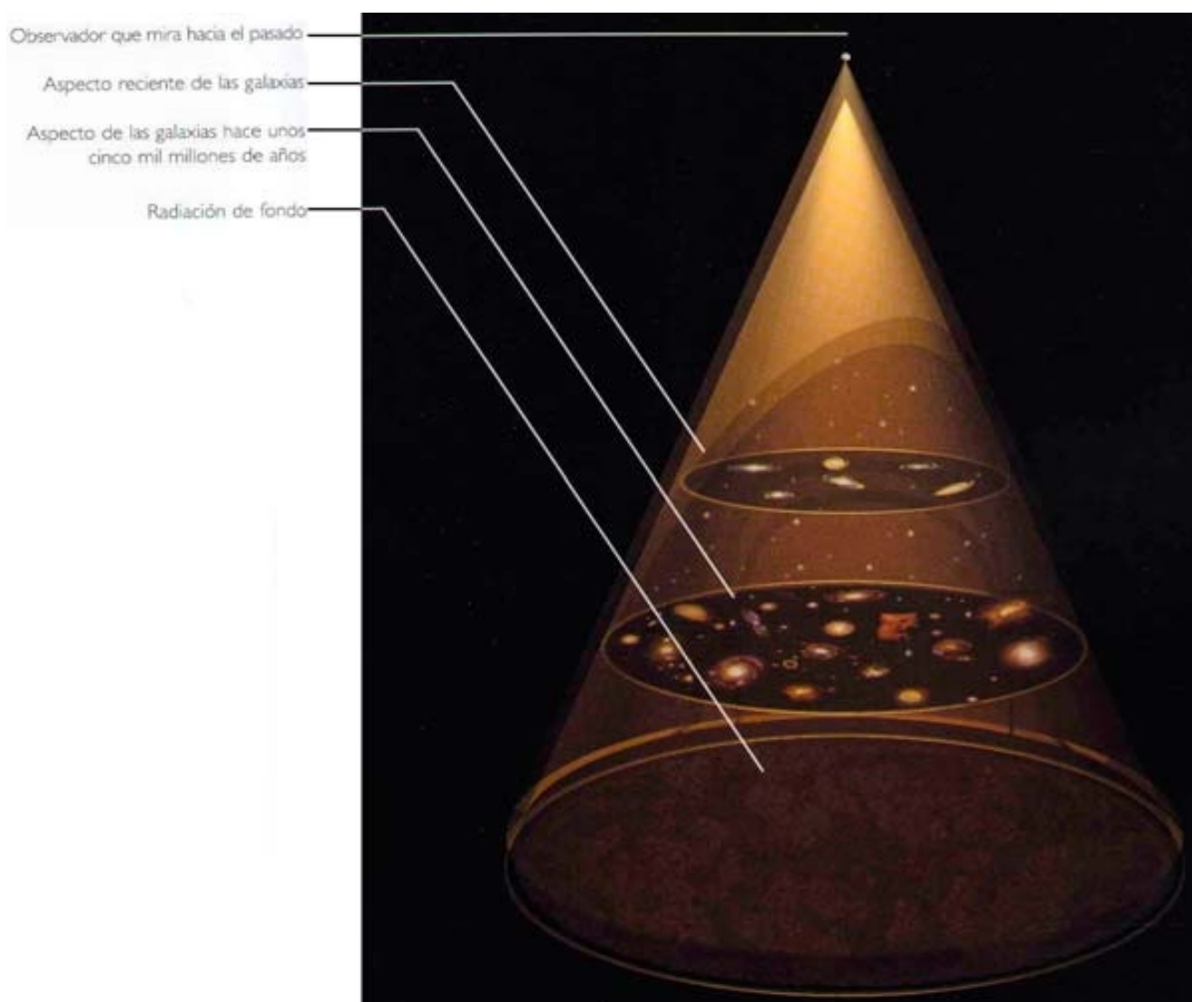
(FIG. 2.5) CONO DE LUZ DEL PASADO
