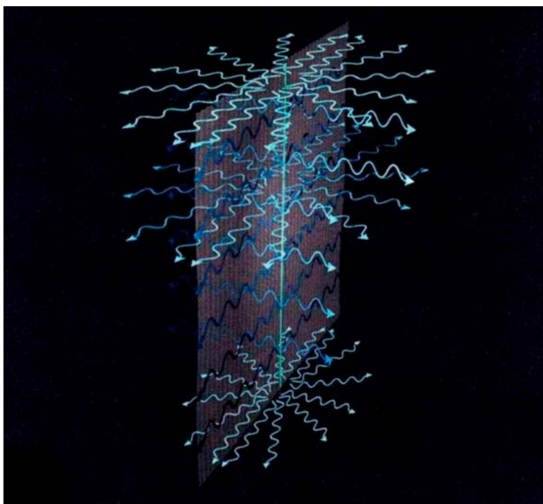
(FIG. 7.15) En el modelo de Randall-Sundrum, las ondas gravitatorias de corta longitud de onda pueden sustraer energía de las fuentes de la membrana, provocando una violación aparente de la ley de conservación de la energía.
