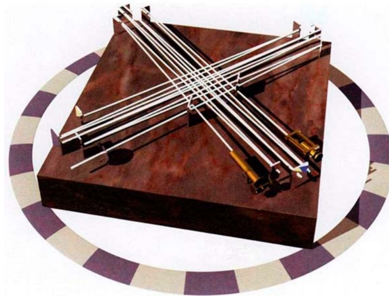
(FIG. 1.3) MIDIENDO LA VELOCIDAD DE LA LUZ
