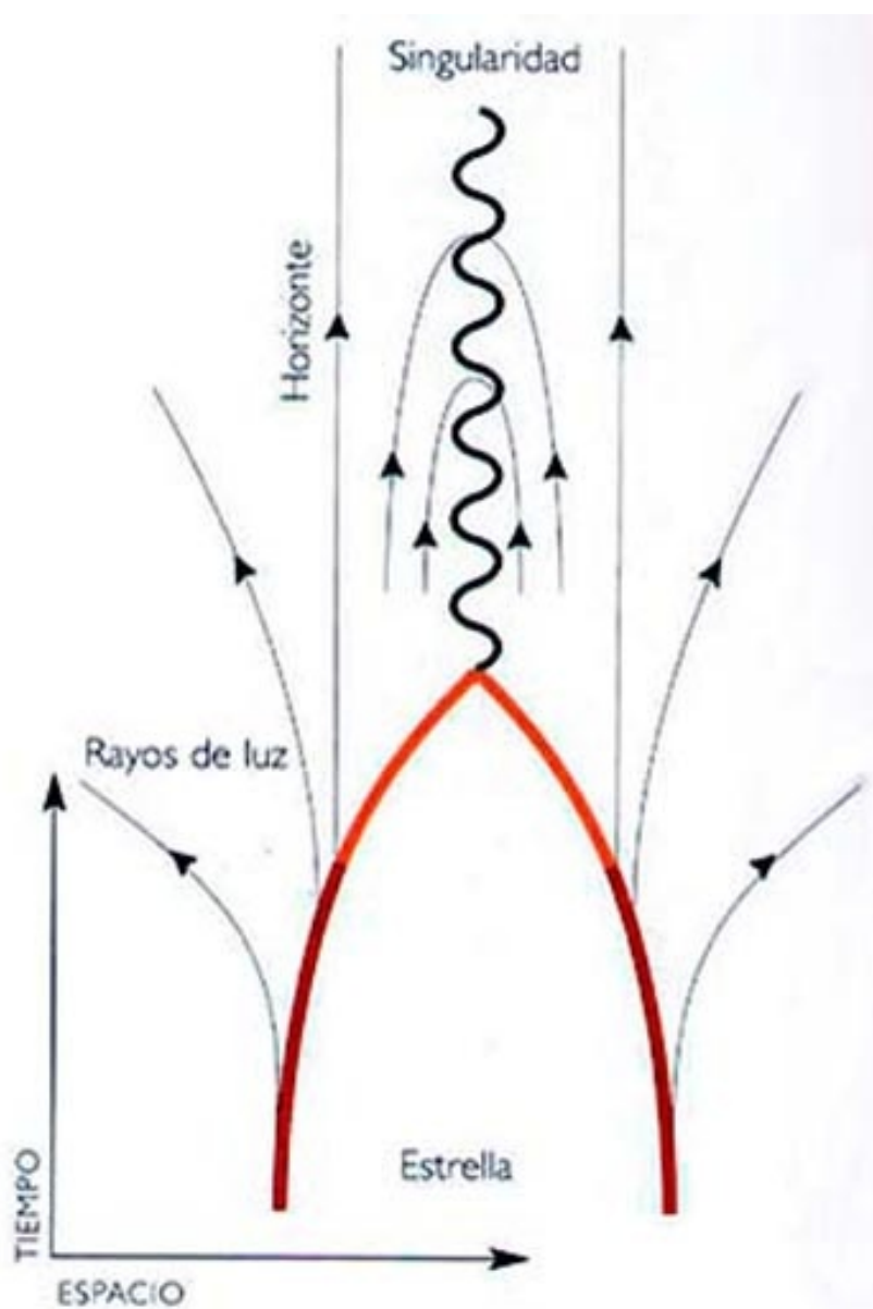
(Fig.4.13) Si la estrella se colapsa (líneas rojas que se cortan en un punto) la deformación deviene tan grande que los rayos de luz de las proximidades de la estrella se mueven hacia adentro. Se ha formado un agujero negro, una región del espacio-tiempo de la cual la luz no puede escapar
