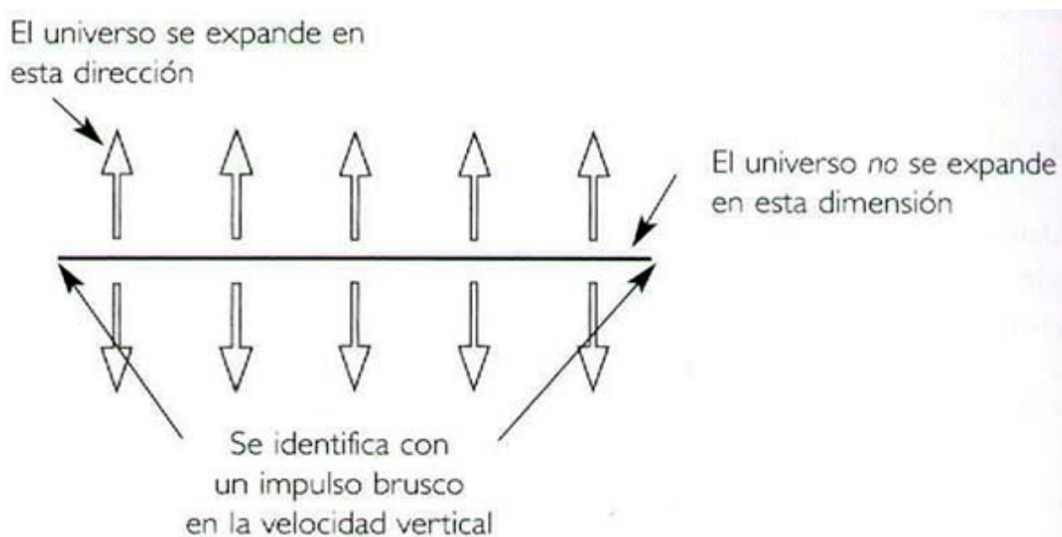
(FIG. 5.18) ESPACIO-TIEMPO DE FONDO CON CURVAS TEMPORALES CERRADAS
