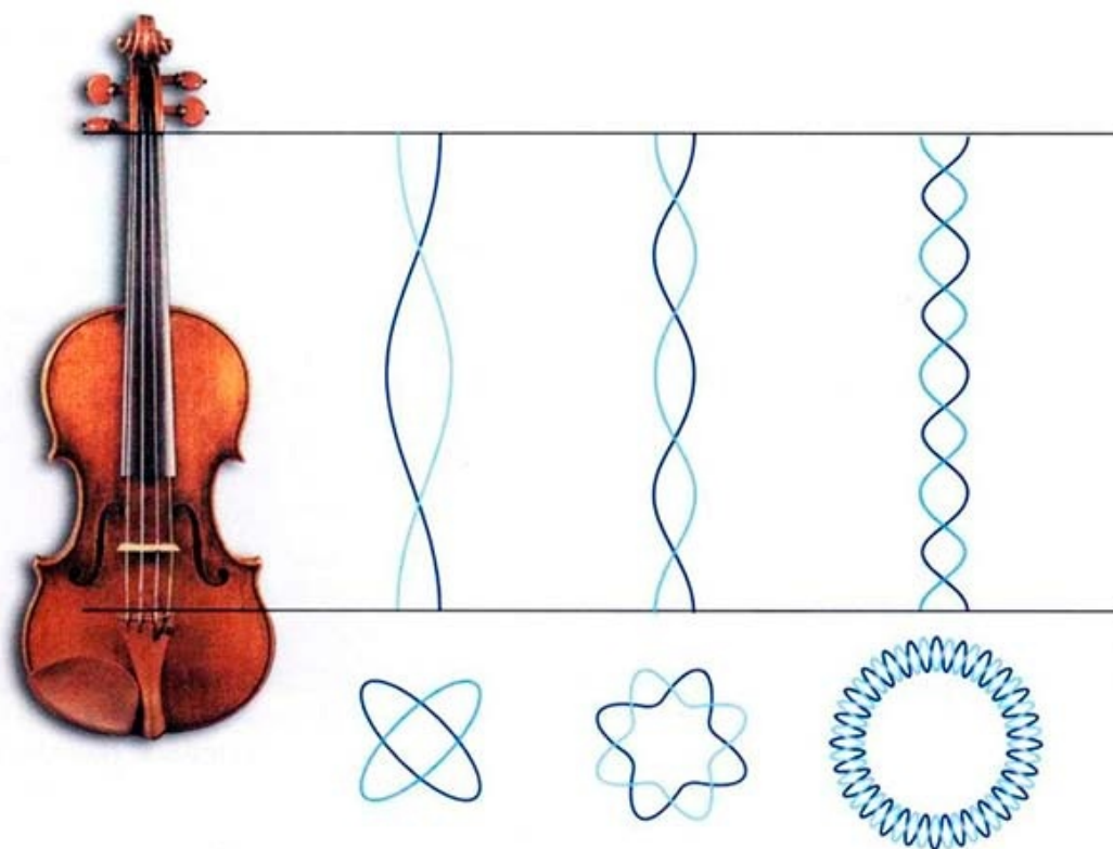
(FIG. 2.14) OSCILACIONES DE CUERDAS
