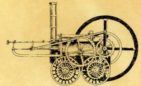
Locomotora a vapor de Trevithick.
